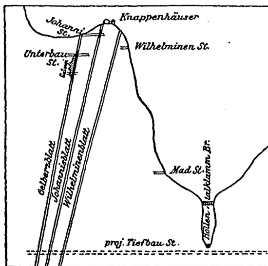
Profil durch das Gangstreichen.
